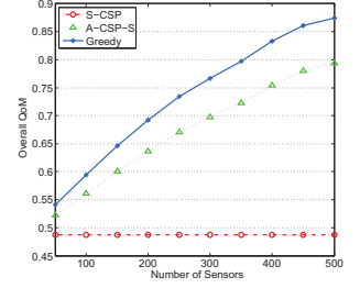
Fig. 4. Greedy vs S-CSP & A-CSP-S
